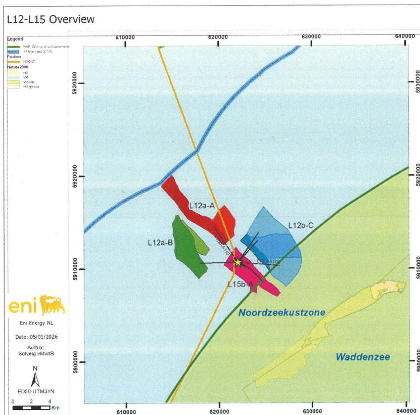
Figuur 1: Overzicht van het L15-FA-1 platform, de voorkomens waaruit aardgas wordt geproduceerd, het Natura 2000-gebied de Noordzeekustzone en de NOGAT-pijpleiding. De doorgetrokken lijnen vanaf het platform betreffen bestaande putten. De gestippelde lijnen betreffen de nieuw aan te boren putten.
