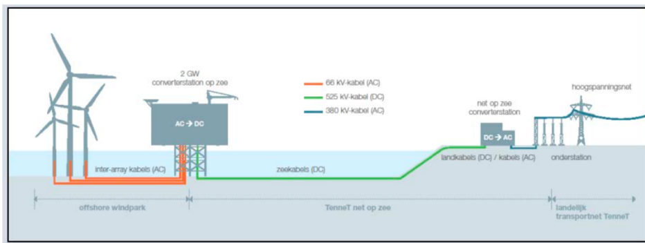
Schematische weergave DC-verbinding (bron: Witteveen en Bos / Royal HaskoningDHV)
